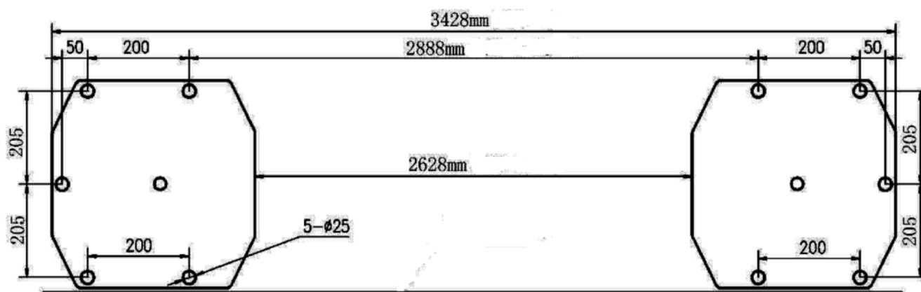
Рис.5 Схема расположения анкерных болтов
